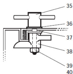
Door fastener Fig. 1
